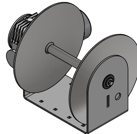
ISOMETRIC VIEW ( N.T.S. )
