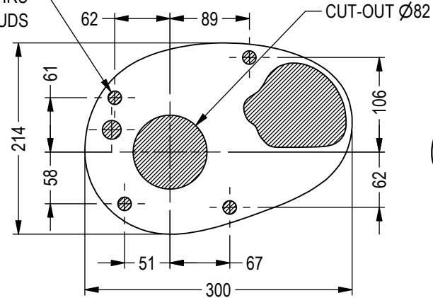
DECK TEMPLATE (N.T.S.)
