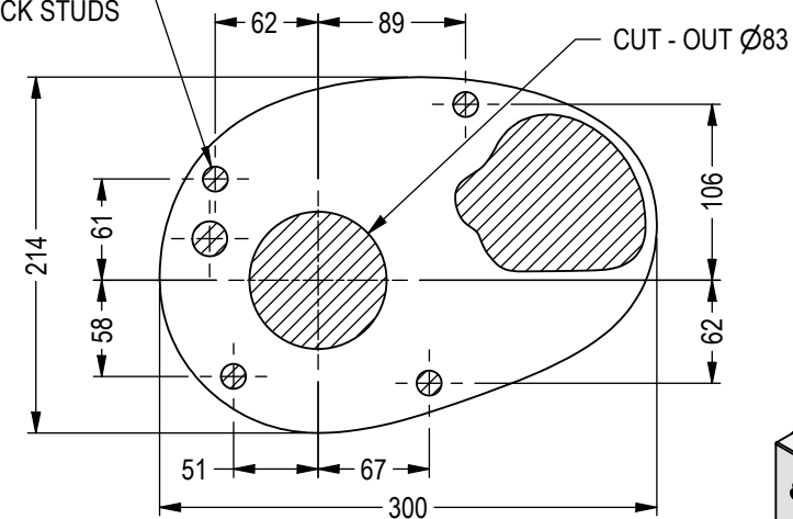
DECK TEMPLATE ( N.T.S. )
