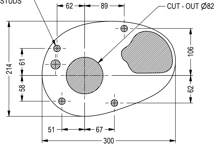
DECK TEMPLATE (N.T.S.)
