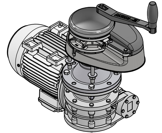
ISOMETRIC VIEW ( N.T.S. )
