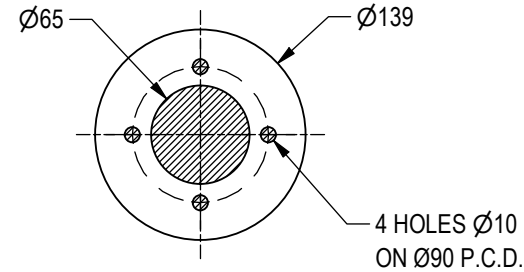
DECK TEMPLATE (N.T.S.)
